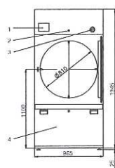
ZEZADU LS 530 680 (PARNÍ MODEL)
