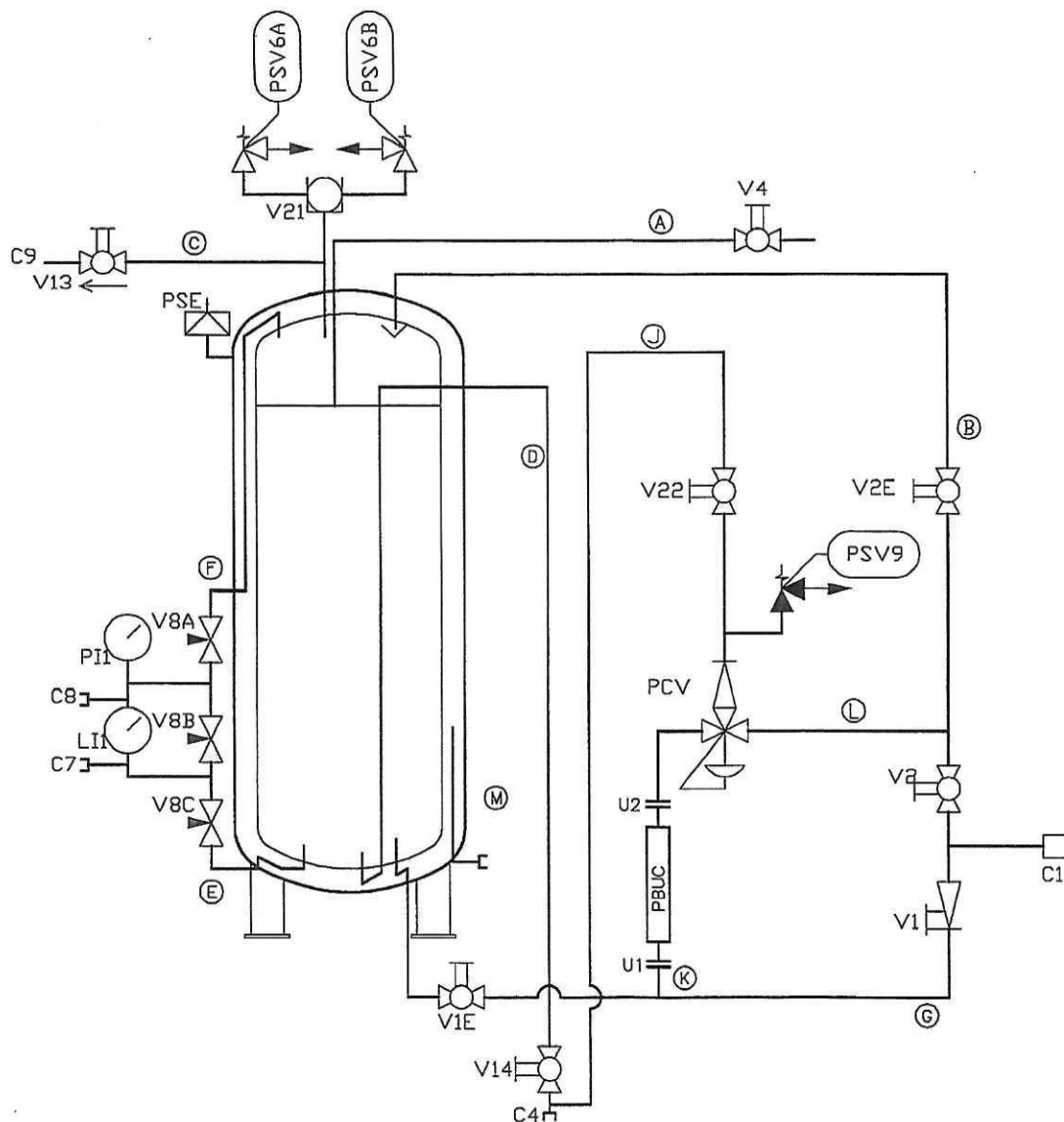
SCHEMA ZAPOJENÍ
